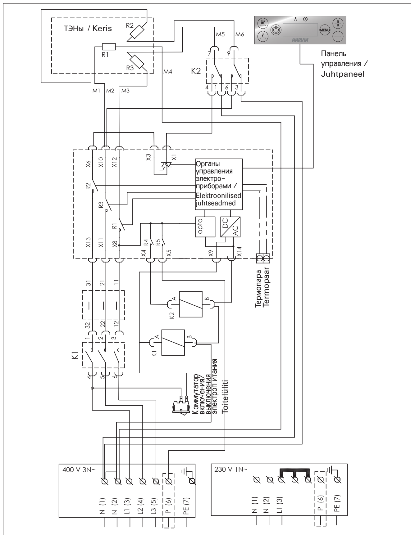
Рис. 12. Электромонтаж каменки
