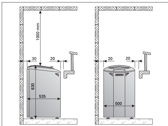
Рис. 9. Расстояния безопасности (мин.) Joonis 9. Kerise miinimum ohutuskauused (mm)
