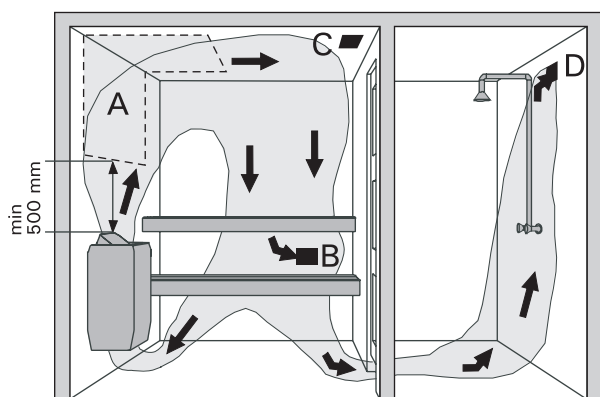
Figure 8. Ventilation du sauna
